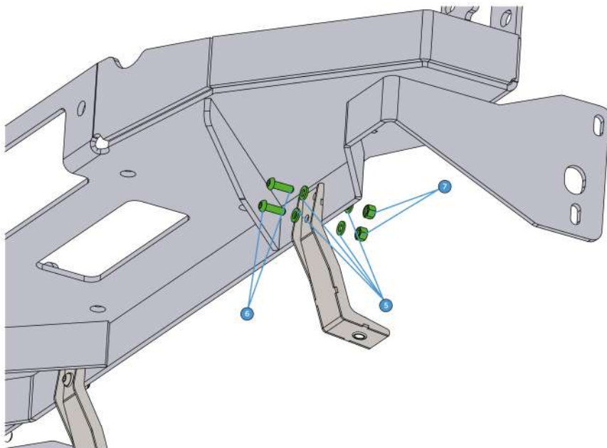
Рисунок 1. Установка кронштейнов бампера
