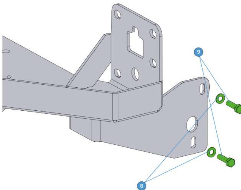
Рисунок 3. Болты M8x30 — крепление к поперечине
