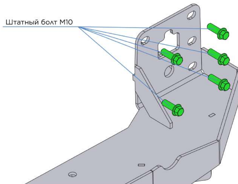
Рисунок 2. Штатные болты M10 в лонжероны
